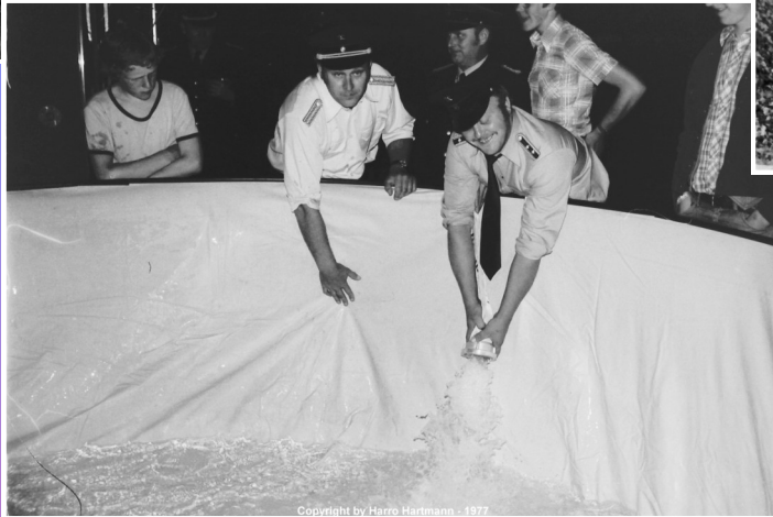
Schlauchbrücke aus Leiterteilen, Fahren im Gelände und Aufbau eines Wasserbehälters.
